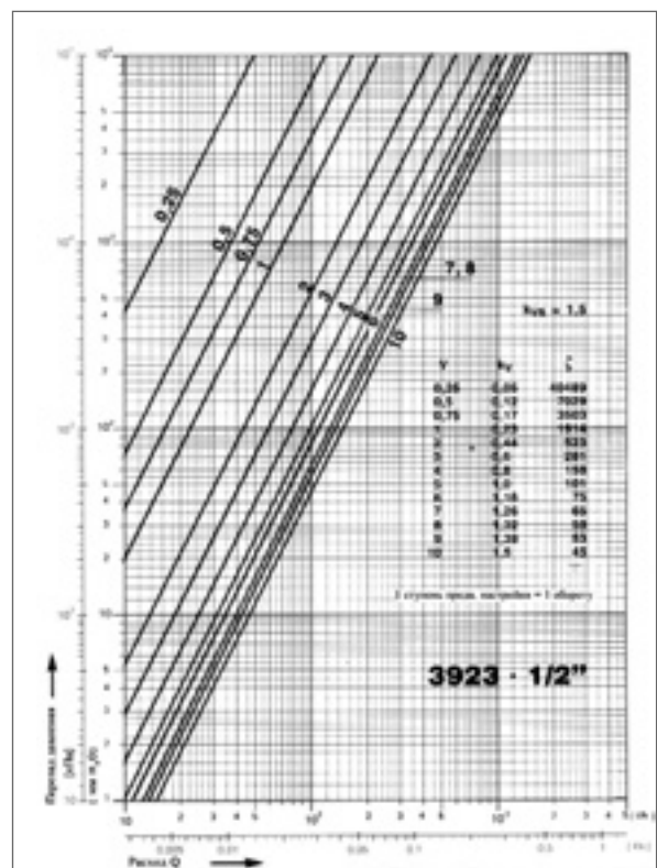
Рис. 36. Номограмма определения настроек обратного вентиля для dP_{в2} и расхода m_p .
