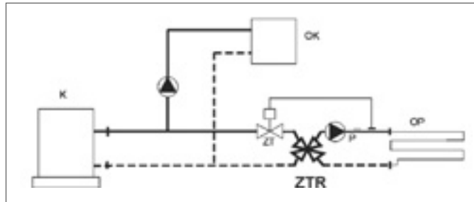
Рис. 6. Схема смесительной системы с полуавтоматическим регулированием: OK - конвективное отопление OP - подпольное отопление P - насос ZT - термостатический вентиль ZTR - четырехходовой вентиль
