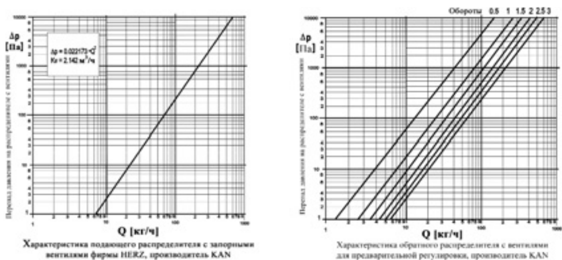
Рис. 41. Характеристика вентилях, встроенных в распределитель.
