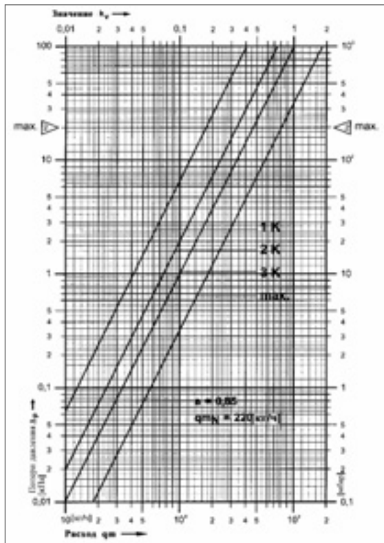
Рис. 35. Номограмма определения dP_{в1} для значения расхода m_p .
